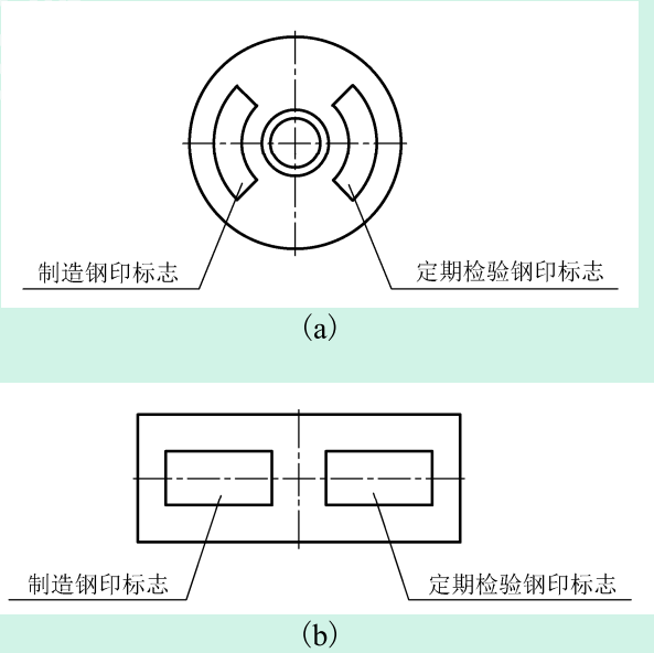
图 D-1 钢印标志位置示意图
